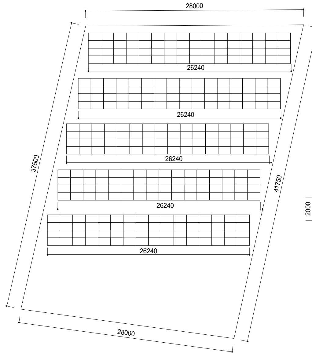
傾斜利用のパネル間2000、全面パネルの影注意・基礎杭にて調整
